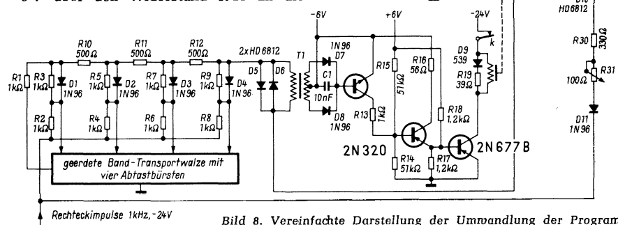
Bild 8. Vereinfachte Darstellung der Umwandlung der Programmierung in eine Drehbewegung eines Schrittelais
