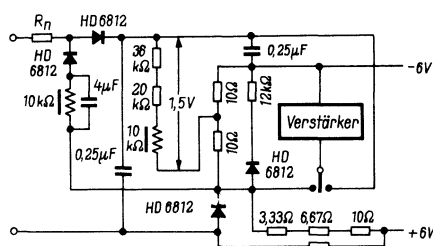
Bild 6. Die Brücke bei Wechselspannungsmessungen
