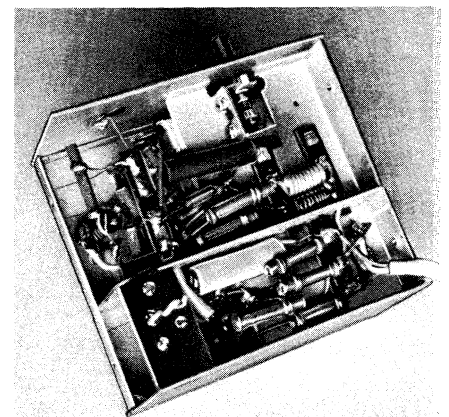
Bild 4. Blick in die Verdrahtung des umgebauten Pendelaudions.
