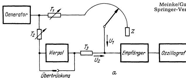
Bild 11 a. Blockschaltung bei der Phasen- und Dämpfungsmessung von Vierpolen
