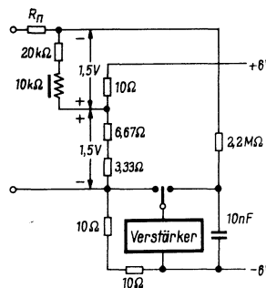
Bild 7. Die Brücke zur Messung von Isolationswiderständen mit Gleichspannung von 500 V
