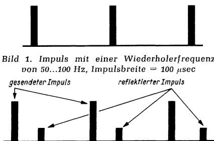
Bild 2. Sendeimpuls mit Echo
