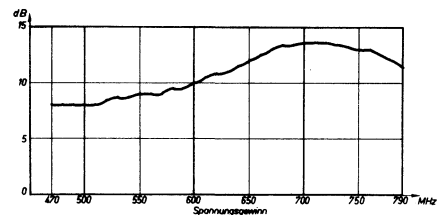
Bild 3. Spannungsgewinn der UHF-Breitbandantenne DFA 1 LM 25
