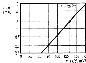
Bild 3. Durchlaßstrom in Abhängigkeit von der Durchlaßspannung
