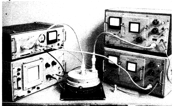
Bild 7. Meßplatz. Links oben: Empfänger, links unten: Oszillograf, rechts oben: Sender, rechts unten: Überlagerungsoszillator
