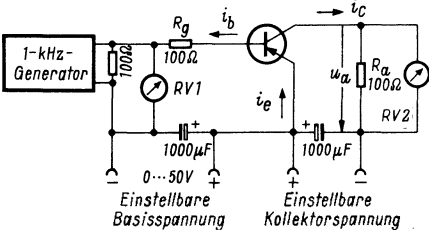
Meßschaltung für die Stromverstärkung \alpha' eines Transistors
